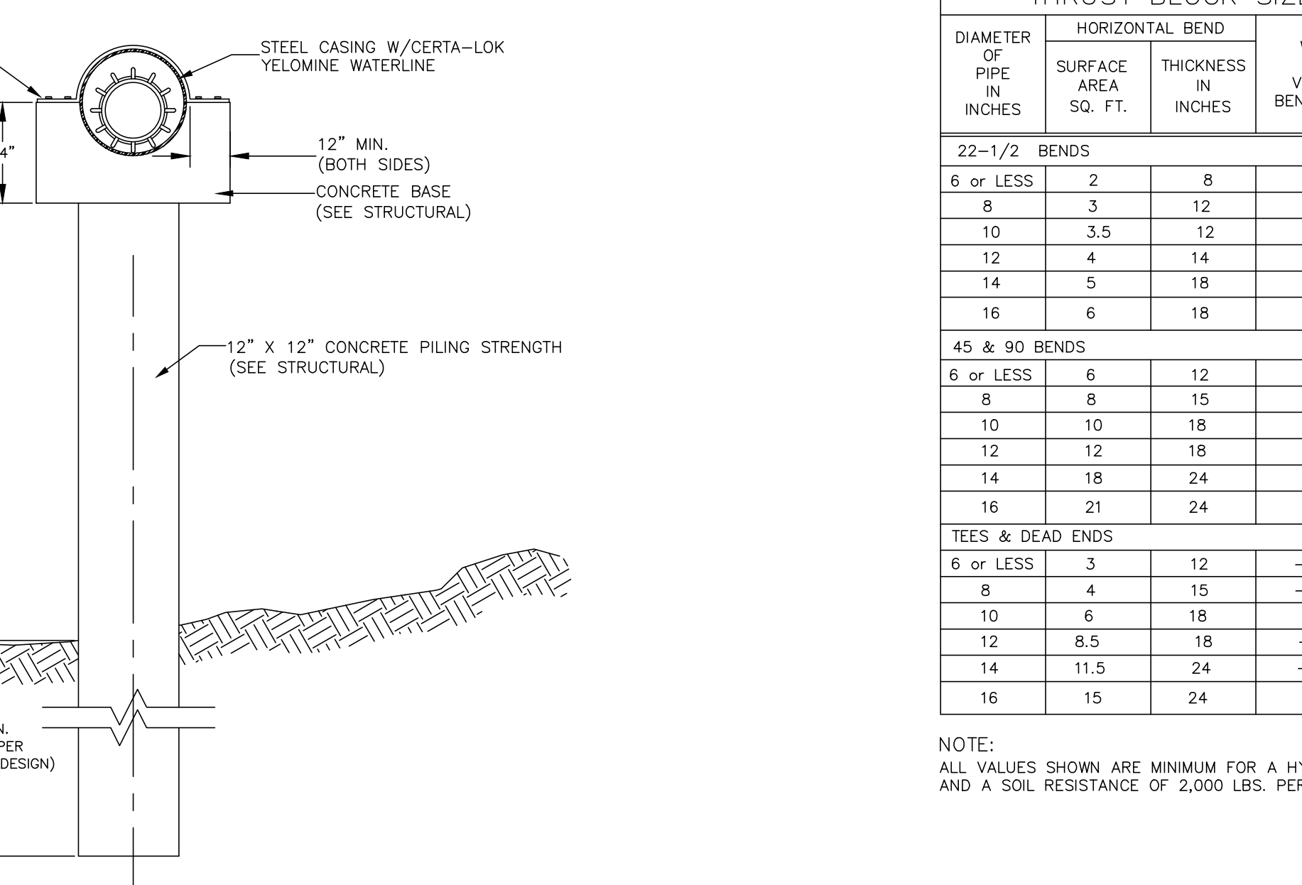
THRUST BLOCKS DETAILS N.T.S.
