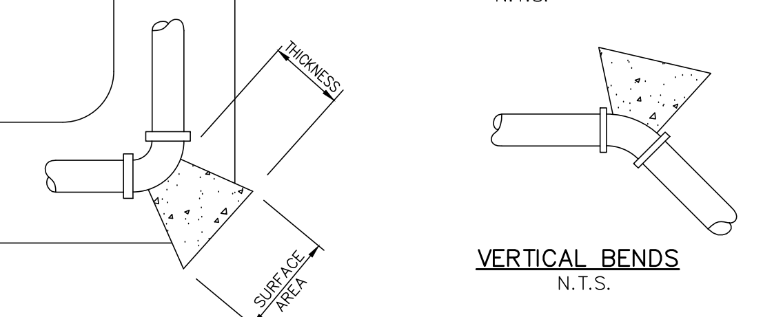
HORIZONTAL BENDS N.T.S.
