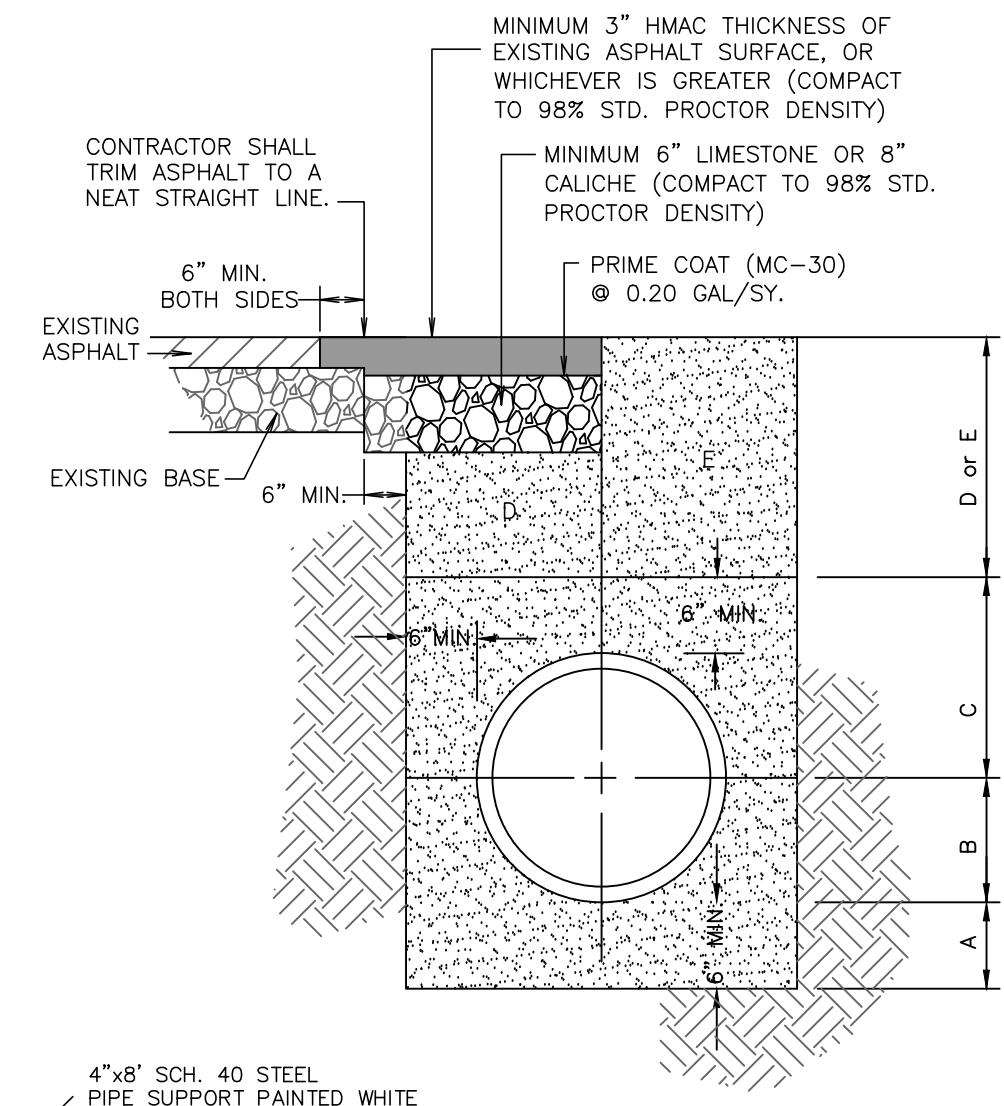
STANDARD PIPE BEDDING N.T.S.
