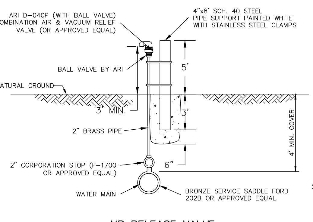
AIR RELEASE VALVE N.T.S.
